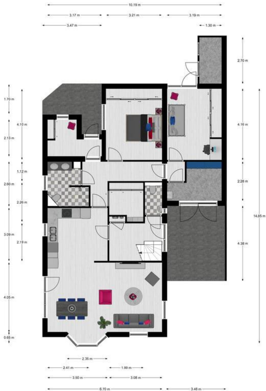
Begane grond, Walstro 3 te Nijverdal De plattegronden zijn geschikt voor promotionele doeleinden. Er kunnen geen rechten aan ontleend worden. © Topr.nl
