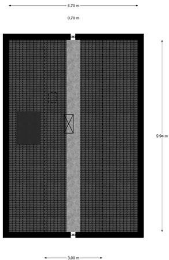
Vliering, Walstro 3 te Nijverdal De plattegronden zijn geschikt voor promotionele doeleinden. Er kunnen geen rechten aan ontleend worden. © Topr.nl
